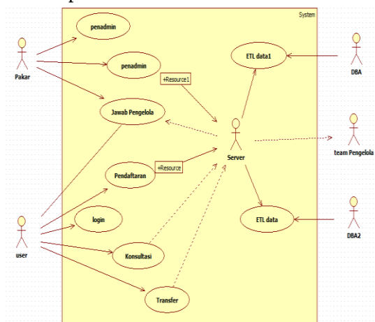
Gambar 4.4. Use Case Diagram Design Interface Jasa Konsultasi Rekam Medis
