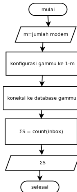
Gambar 6. Sinkronisasi Data Inbox
