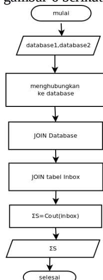
Gambar 5. Sinkronisasi Antar Database
