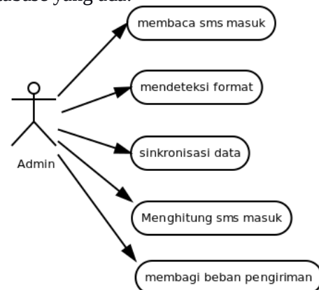
Gambar 7 Use Case Aplikasi
