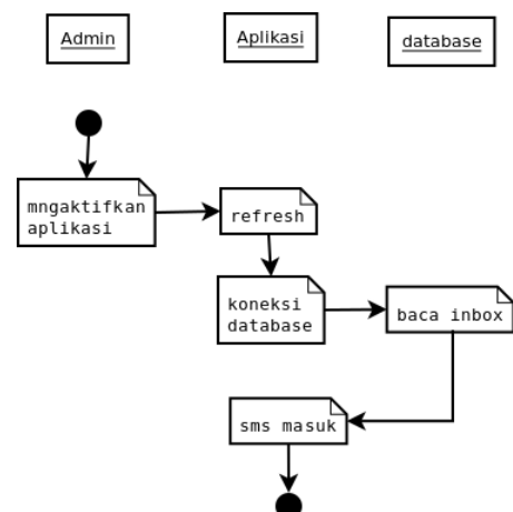
Gambar 8. Activity Diagram Pembacaan SMS Masuk
