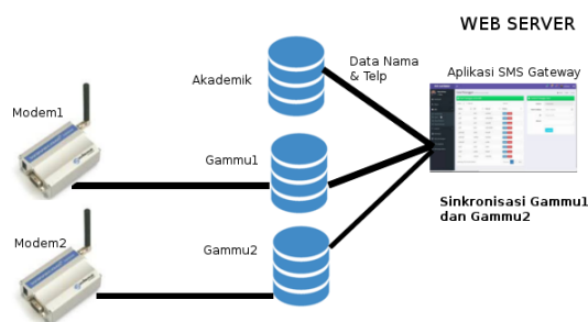
Gambar 2. Topologi Sistem Sinkronisasi dengan banyak Database
