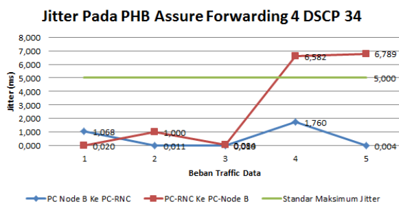
Gambar 10 Grafik Jitter Pada PHB Assure Forwarding 4 Dengan Beban Traffic Data 1-5
