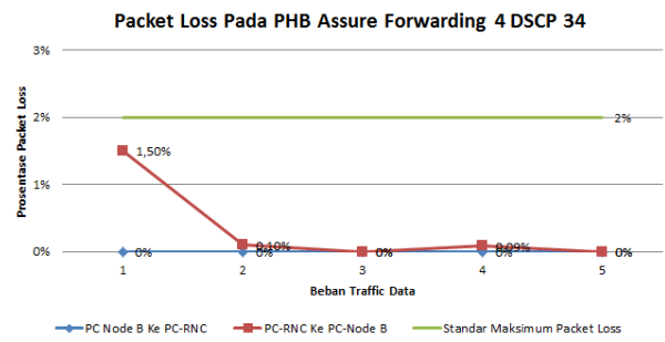
Gambar 16 Grafik Packet Loss Pada PHB Assure Forwarding 4 Dengan Beban Traffic Data 1-5
