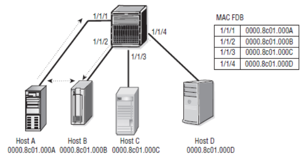
Gambar 2 Prinsip Kerja Switch
