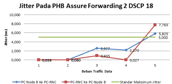
Gambar 8 Grafik Jitter Pada PHB Assure Forwarding 2 Dengan Beban Traffic Data 1-5
