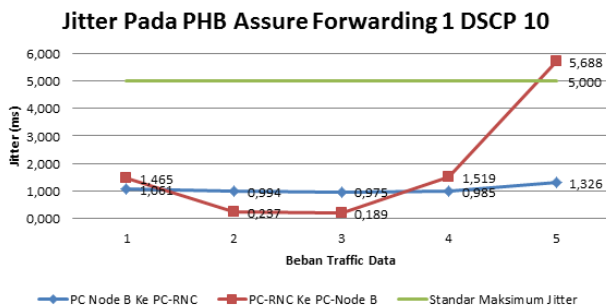
Gambar 7 Grafik Jitter Pada PHB Assure Forwarding 1 Dengan Beban Traffic Data 1-5
