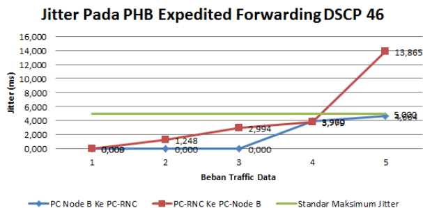
Gambar 11 Grafik Jitter Pada PHB Expedited Forwarding Dengan Beban Traffic Data 1-5
