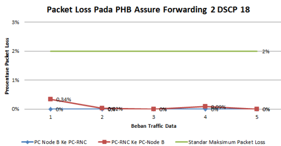
Gambar 14 Grafik Packet Loss Pada PHB Assure Forwarding 2 Dengan Beban Traffic Data 1-5
