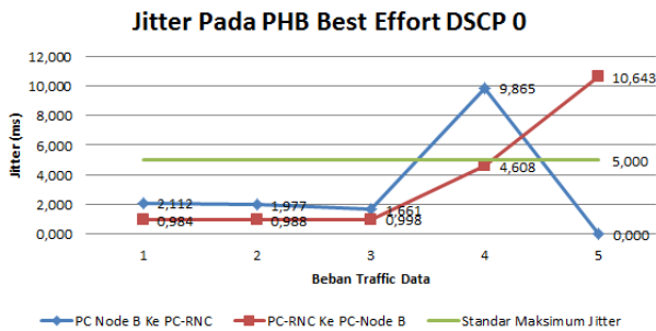
Gambar 6 Grafik Jitter Pada PHB Best Effort Dengan Beban Traffic Data 1-5
