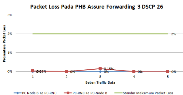
Gambar 15 Grafik Packet Loss Pada PHB Assure Forwarding 3 Dengan Beban Traffic Data 1-5
