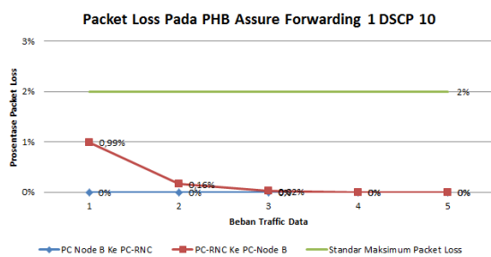
Gambar 13 Grafik Packet Loss Pada PHB Assure Forwarding 1 Dengan Beban Traffic Data 1-5
