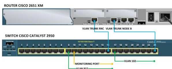
Gambar 4 Koneksi Fisik Pada Jaringan Pengujian (Testbed)
