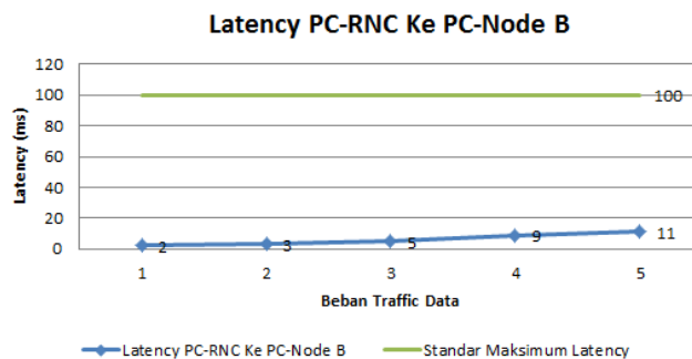
Gambar 20 Grafik Nilai Latency Dari PC-RNC Menuju PC-Node B
