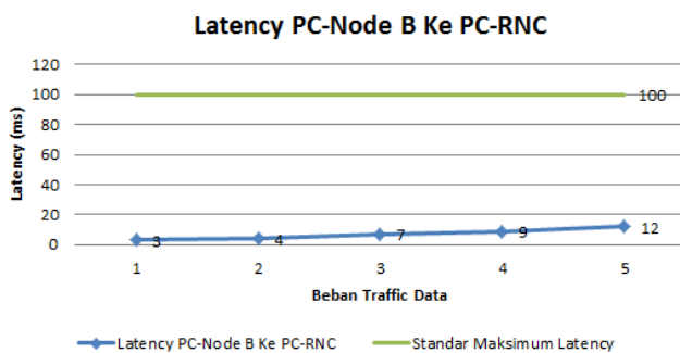
Gambar 18 Grafik Nilai Latency Dari PC-Node B Menuju PC-RNC
