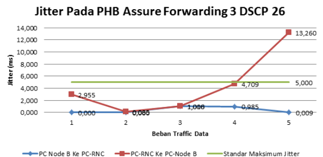
Gambar 9 Grafik Jitter Pada PHB Assure Forwarding 3 Dengan Beban Traffic Data 1-5
