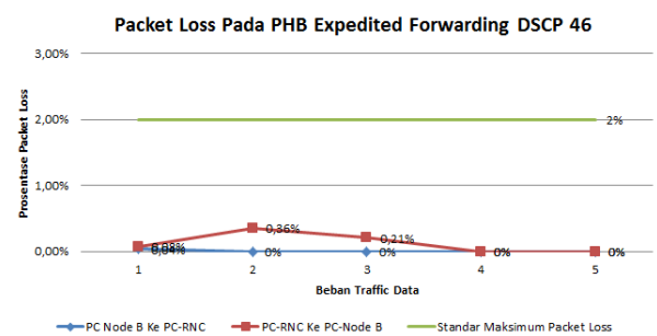
Gambar 17 Grafik Packet Loss Pada PHB Expedited Forwarding Dengan Beban Traffic Data 1-5
