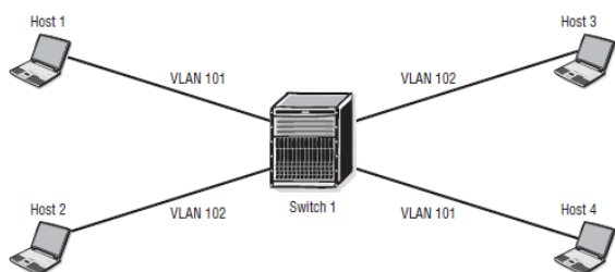
Gambar 3 Penugasan VLAN pada switch
