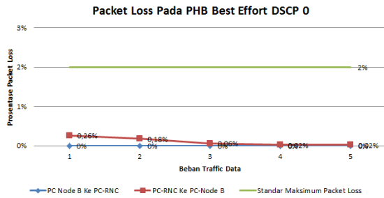
Gambar 12 Grafik Packet Loss Pada PHB Best Effort Dengan Beban Traffic Data 1-5
