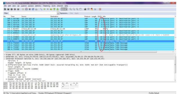
Gambar 5 Hasil Proses Packet Capture Melalui PC-Monitoring Dengan Aplikasi Wireshark
