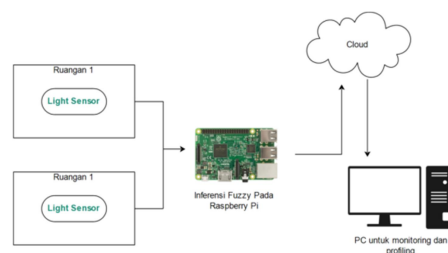
Gambar 1 Arsitektur Sistem
