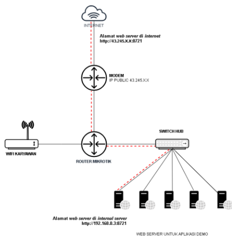
Gambar 1. Topologi Jaringan Sekawan Media
