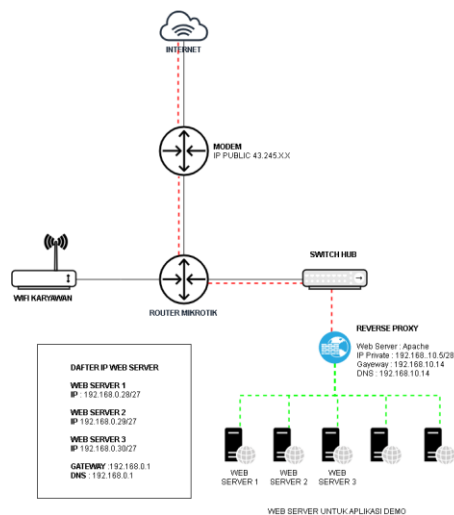
Gambar 3. Topologi Jaringan Yang Disarankan
