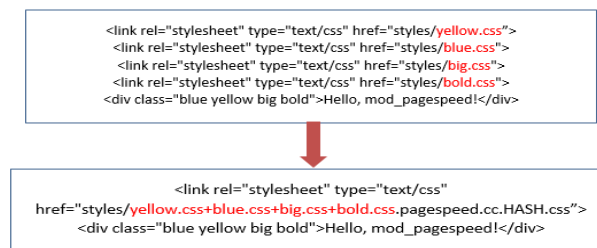
Gambar 3 Proses Kombinasi Beberapa File CSS Oleh Pagespeed
