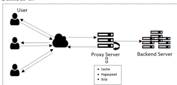
Gambar 1. Topologi Cara Kerja Server Reverse Proxy
