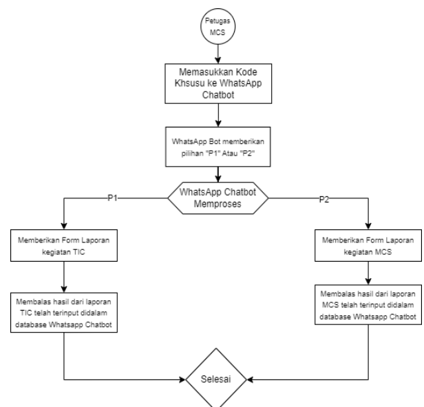
Gambar 7. Diagram Activity Petugas lapangan dengan Chatbot
