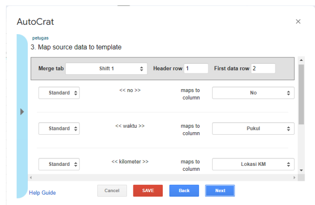
Gambar 4. Configurasi Autocrat untuk membuat Mail merge
