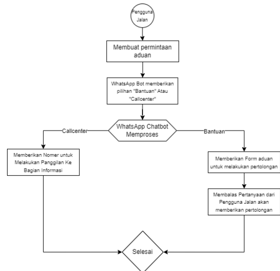
Gambar 6. Diagram Activity Pengguna Jalan dengan Chatbot
