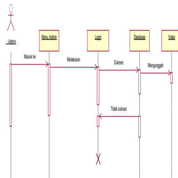
Gambar 8. Sequence Diagram Mengunggah Video
